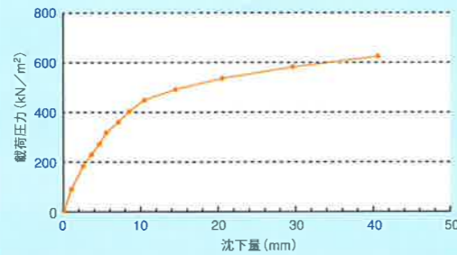
載荷圧力-沈下量曲線の結果例
